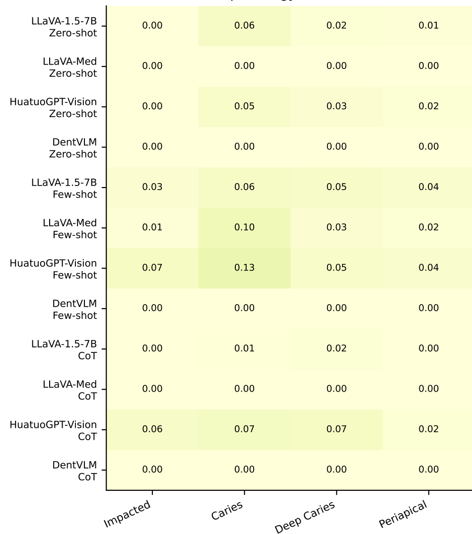
DENTEX pathology F1 (one-vs-rest)
