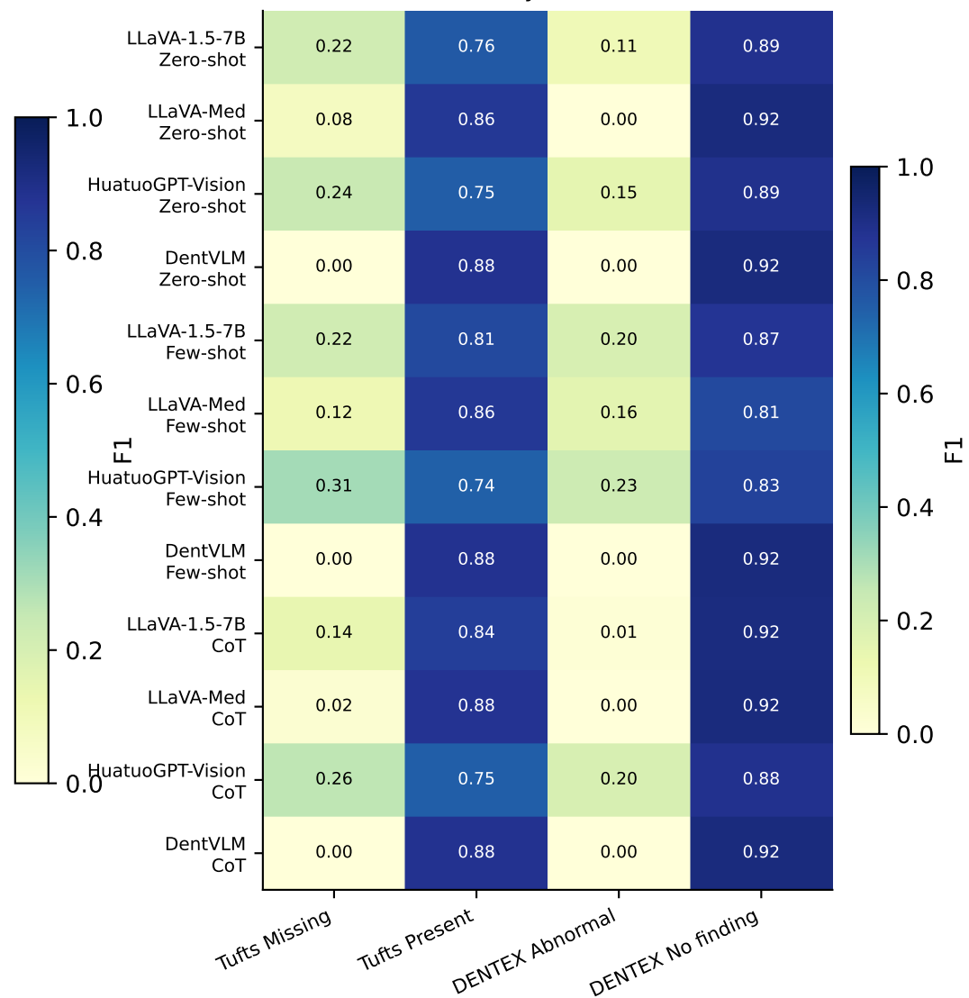
Binary-task F1
